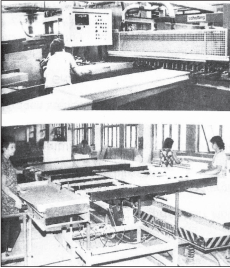
Moderne Trennsäge zur Aufteilung beschichteter Platten auf Bauteilgröße (oben). Anlage zur rationellen Verpackung der Möbelkollis (unten), um 1985
