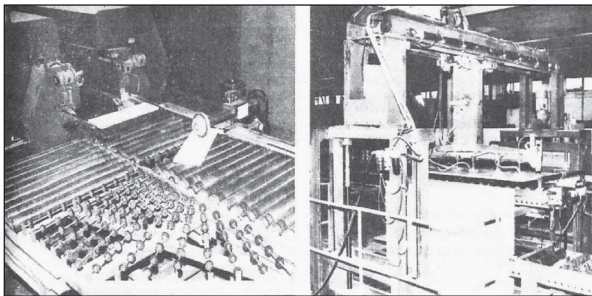
Drehstation und Stapelvorrichtung aus dem eigenen Rationalisierungsmittelbau des VEB Holzindustrie Halberstadt, um 1985.
